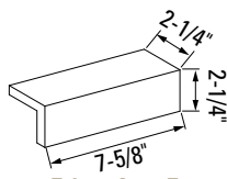
Edge Cap E
